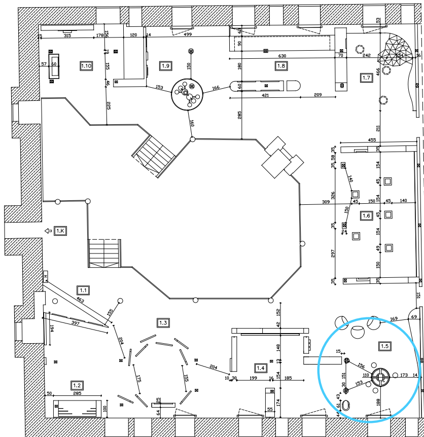
RZUT POZIOMU +1
