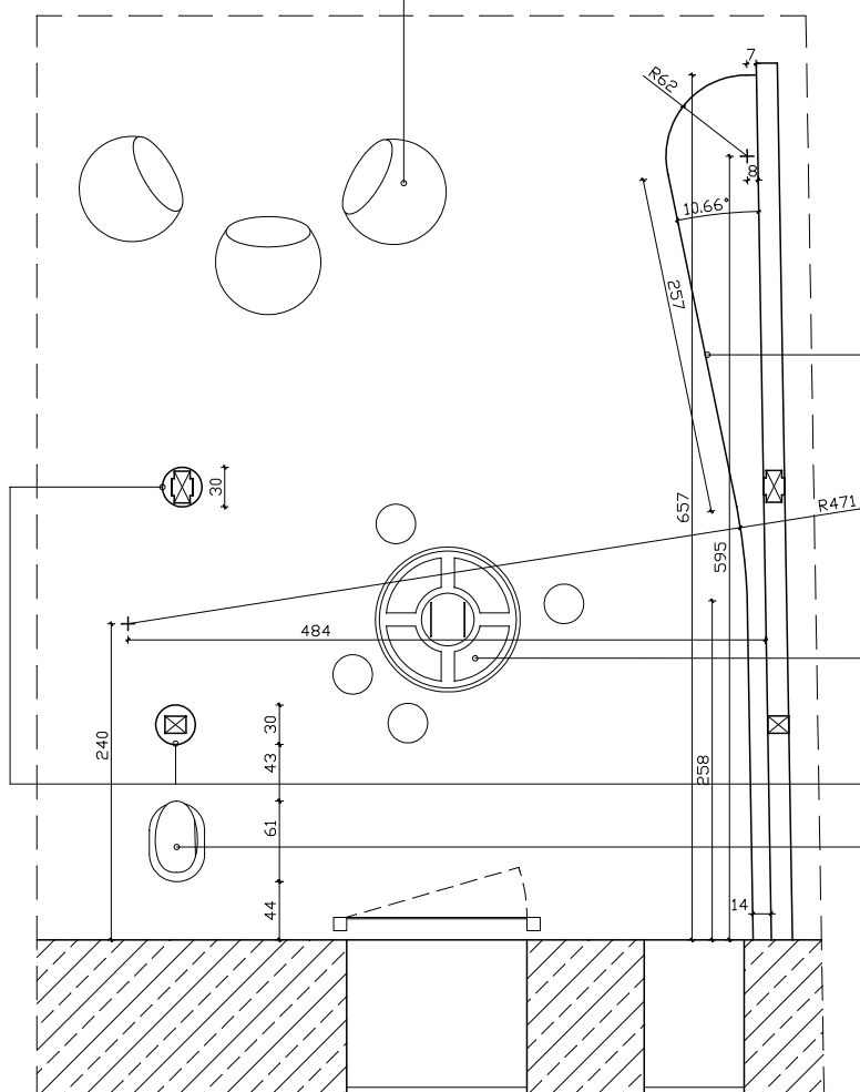
RZUT SYTUACYJNY 1.5
