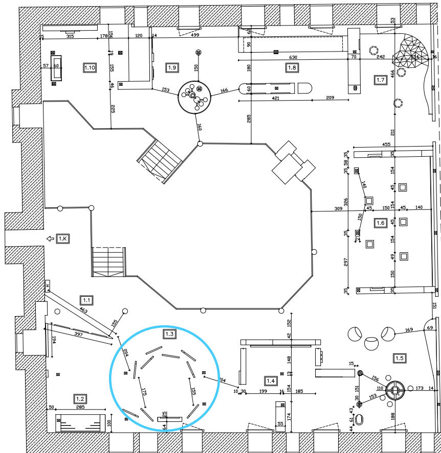
RZUT POZIOMU +1
